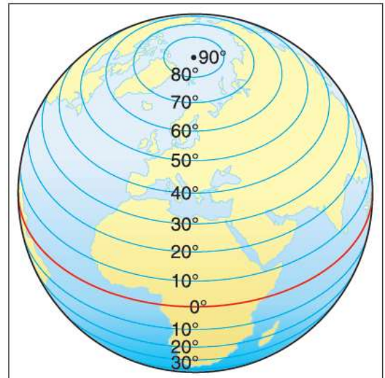
Paraleller
