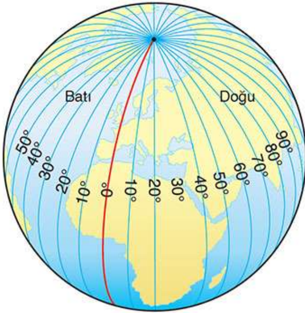
Meridyenlerin Özellikleri
